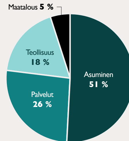
Kuva 7. Lämmityksen päästöjen jakautuminen kulutussektoreittain vuonna 2018 Varsinais-Suomessa. (Hinku-laskenta, SYKE)
