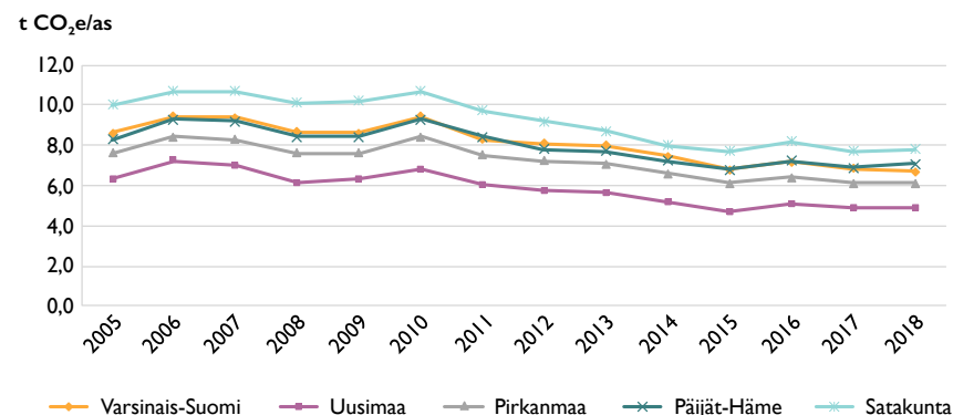
Kuva 3. Varsinais-Suomen ja lähimaakuntien ilmastopäästöjen kehitys 2005–2018 asukasta kohden (t CO 2 e/as). (Hinku-laskenta, SYKE)
