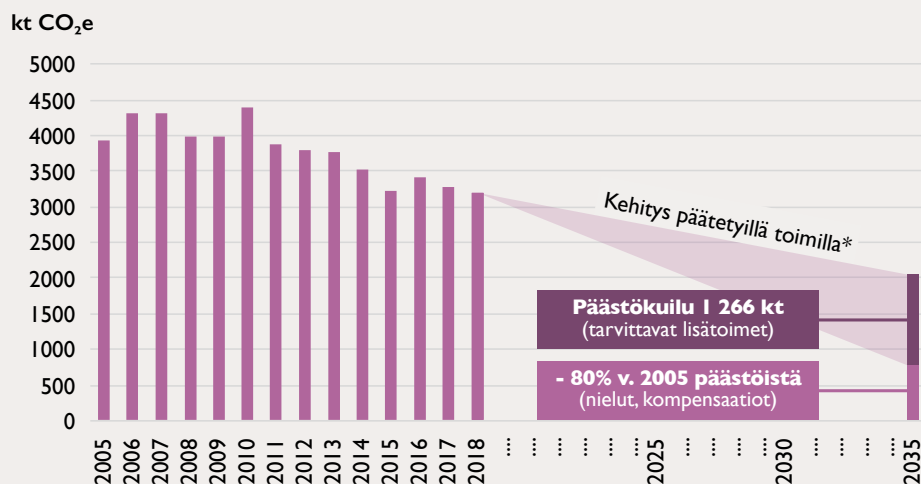
Kuva 4. Varsinais-Suomen päästökaikitys (kt CO 2 e) 2005–2018 ja polku hiilineutraaliuteen 2035 sekä arvio päästökuilusta. (Hinku-laskenta, SYKE)
