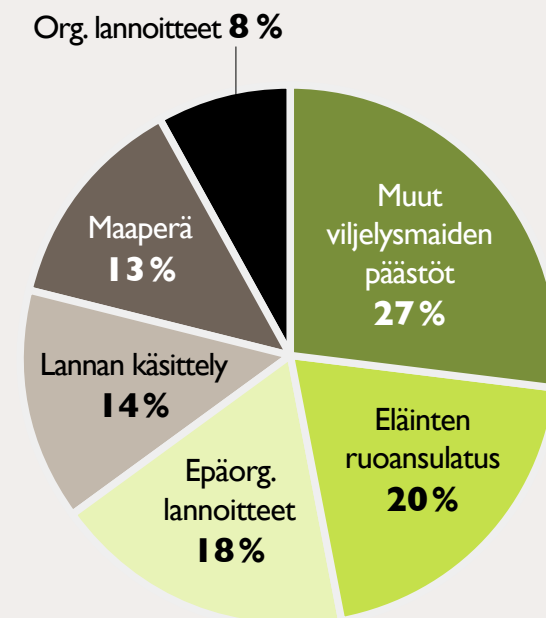
Kuva 9. Maatalouden ilmastopäästöjen jakautuminen vuonna 2018 Varsinais-Suomessa. (Hinku-laskenta, SYKE)
