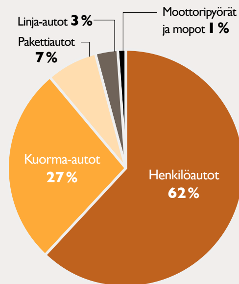
Kuva 8. Tieliikenteen ilmastopäästöjen jakautuminen vuonna 2018 Varsinais-Suomessa. (Hinku-laskenta, SYKE)
