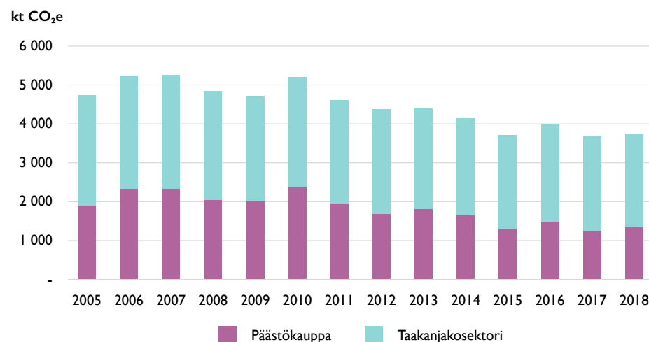
Kuva 1. Varsinais-Suomen päästökauppa- ja taakanjakosektorin päästöjen kehitys (tuhatta hiilidioksidiekvivalenttitonnia, kt CO 2 e) vuosina 2005–2018. (ALas-laskenta, SYKE)
